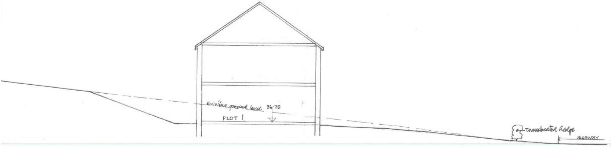
DATUM 34.00 SECTION B-B
